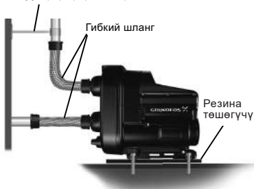
7-сүрөт. SCALA2 үчүн ызы-чууну азайтуу боюнча иш-чаралар
