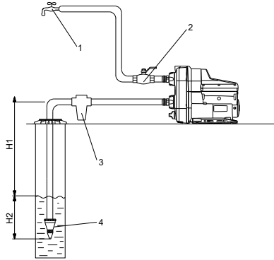
Նկար 9 Ջրի մատակարարումը ջրհորից/ հորանցքից
