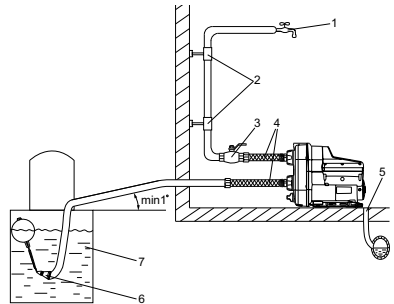
Նկար 10 Ջրի մատակարարումը ռեզերվուարից
