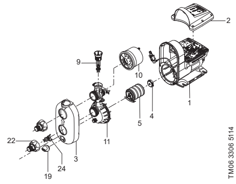
Նկար 2 SCALA2-ի կառուցվածք
